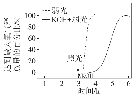
乙 衣藻细胞的氧气释放情况
